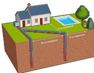
FIGURE 73. SCHÉMA D'UN CAPTAGE VERTICAL AVEC POMPE À CHALEUR (©GÉOTHERMIE-PERSPECTIVES.FR, ADEME-BRGM)
