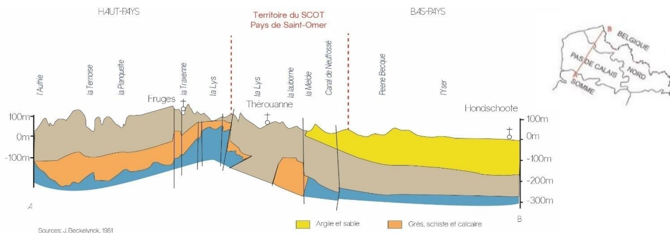
FIGURE 1. COUPE GÉOLOGIQUE SIMPLIFIÉE SUD-OUEST/NORD-EST
