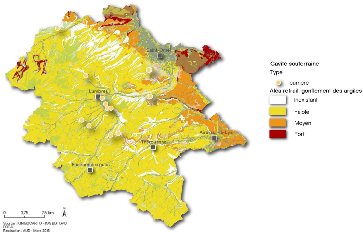
FIGURE 106. SENSIBILITE RETRAIT-GONFLEMENT DES ARGILES
