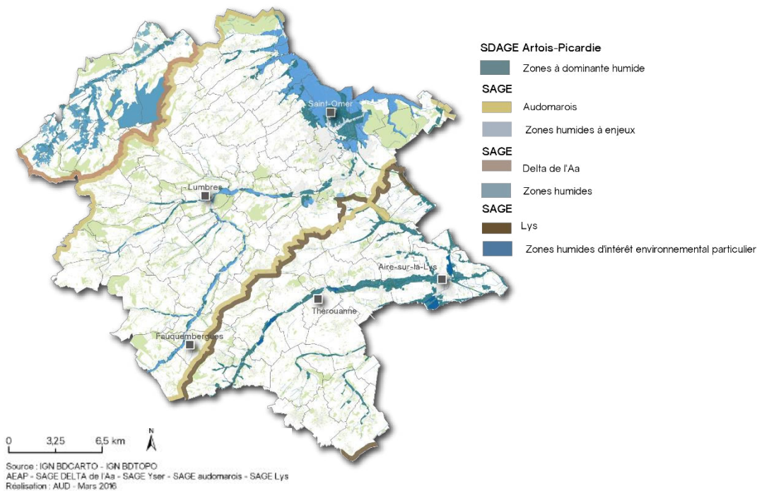
FIGURE 22. ZONES HUMIDES IDENTIFIÉES PAR LE SCHÉMA DIRECTEUR D'AMÉNAGEMENT ET DE GESTION DES EAUX DU BASSIN ARTOIS PICARDIE ET PAR LES SCHÉMAS D'AMÉNAGEMENT ET DE GESTION DES EAUX
