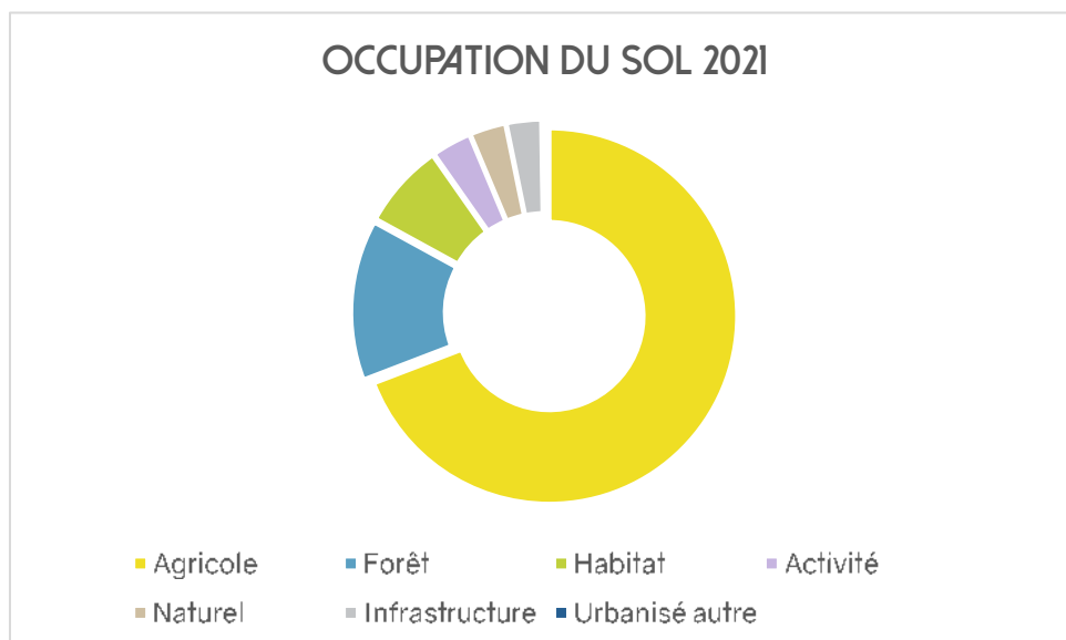
FIGURE 8. OCCUPATION DES SOLS EN 2021
