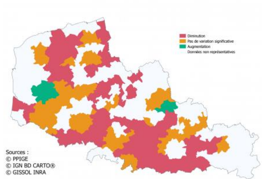
FIGURE 18. ÉVOLUTION DE LA PROPORTION DE CARBONE ORGANIQUE DANS LES SOLS ENTRE 1990 ET 2005, EXEMPLE DE LA PERTE DE RICHESSE
