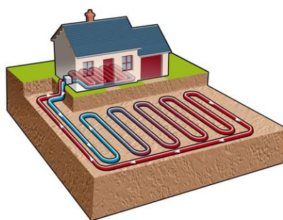
FIGURE 74. SCHÉMA D'UN CAPTAGE HORIZONTAL AVEC POMPE À CHALEUR (©GÉOTHERMIE-PERSPECTIVES.FR, ADEME-BRGM)
