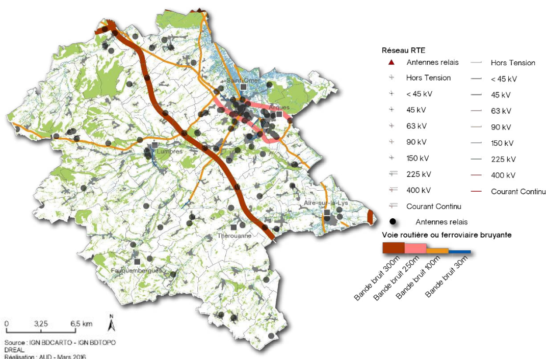
FIGURE I03. ONDES SONORES ET ÉLECTROMAGNÉTIQUES
