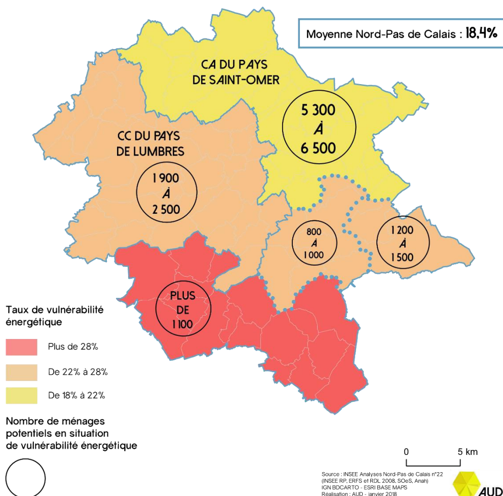
FIGURE 101 : TAUX DE VULNÉRABILITÉ ÉNERGÉTIQUE
