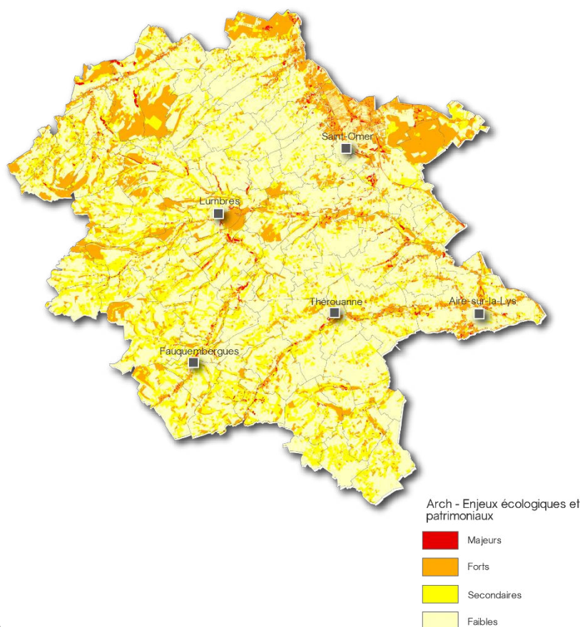
FIGURE 34. ENJEUX ÉCOLOGIQUES ET PATRIMONIAUX
