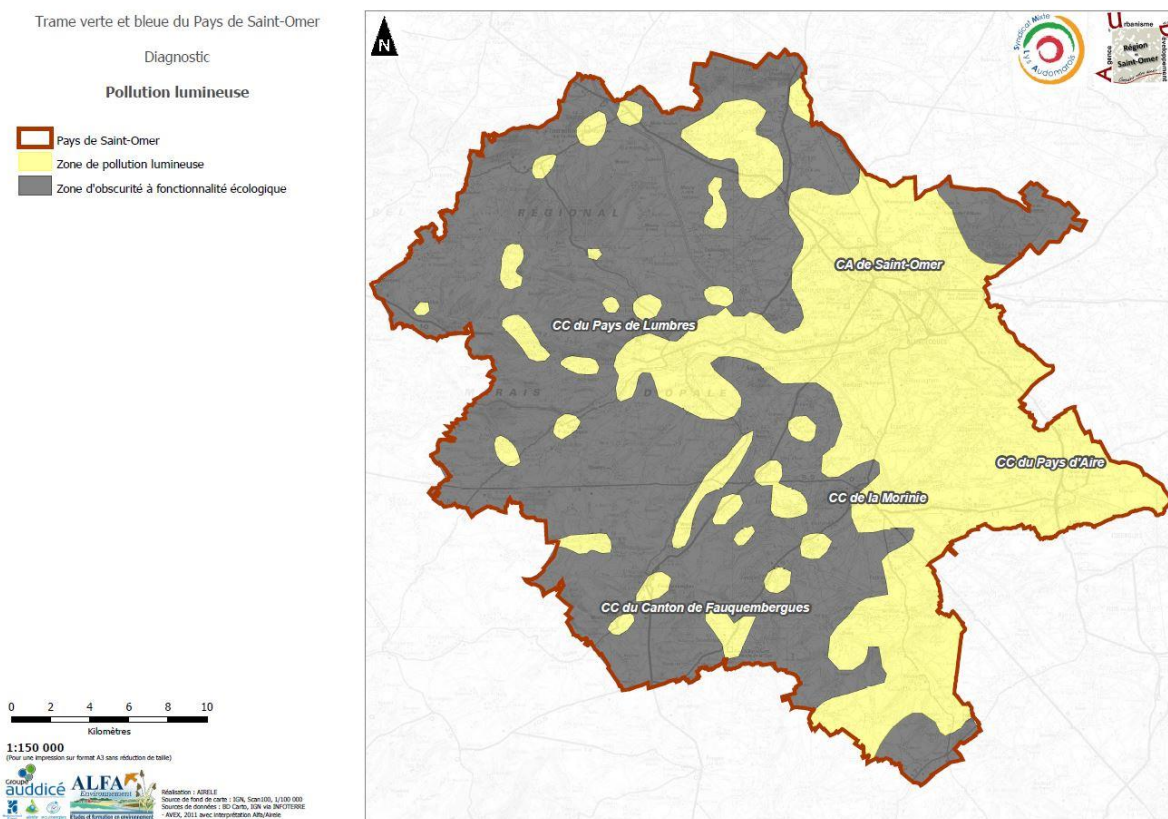
FIGURE 43. POLLUTION LUMINEUSE SUR LE PAYS DE SAINT-OMER
