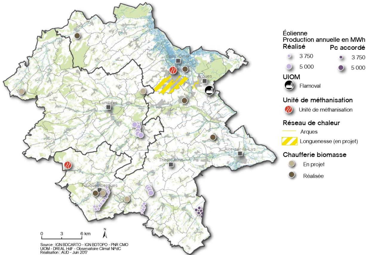
FIGURE 70. RÉPARTITION SUR LE TERRITOIRE DES INSTALLATIONS DE PRODUCTION D'ÉNERGIE RENOUVELABLE ET DE RÉCUPÉRATION HORS SOLAIRE
