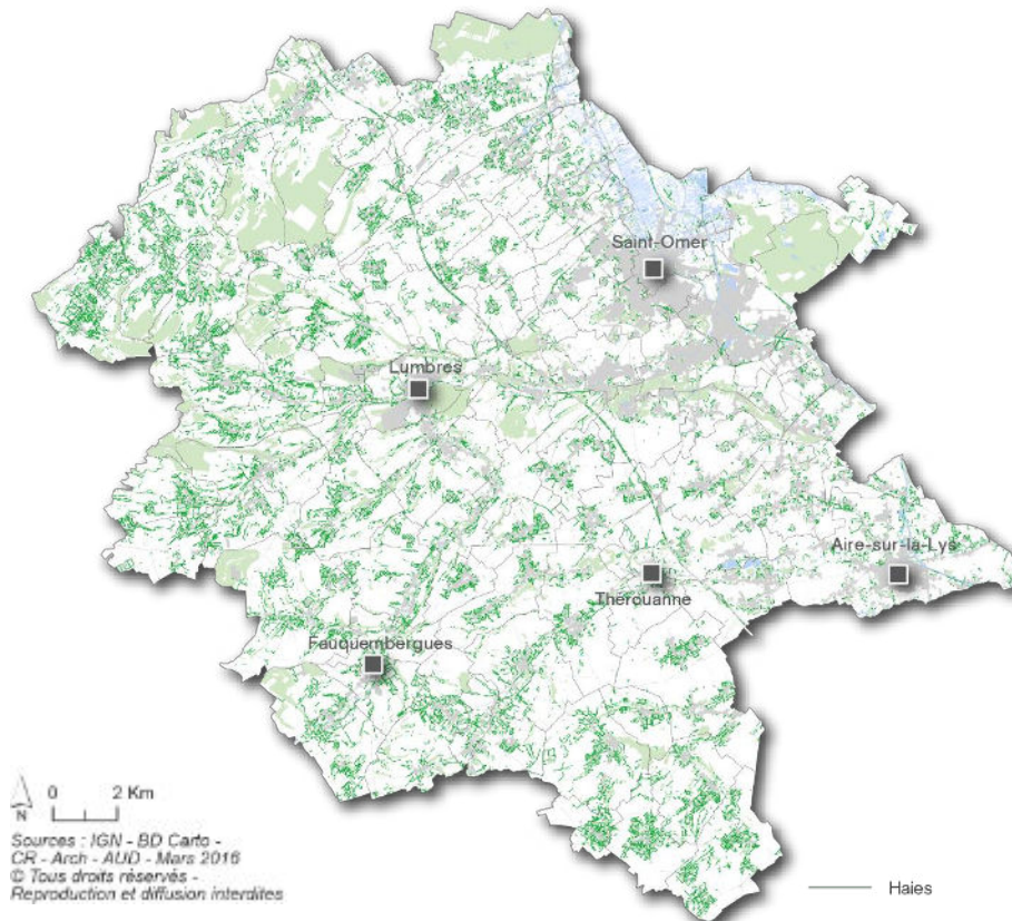
FIGURE 77. LES HAIES BOCAGÈRES SUR LE TERRITOIRE DU SCOT
