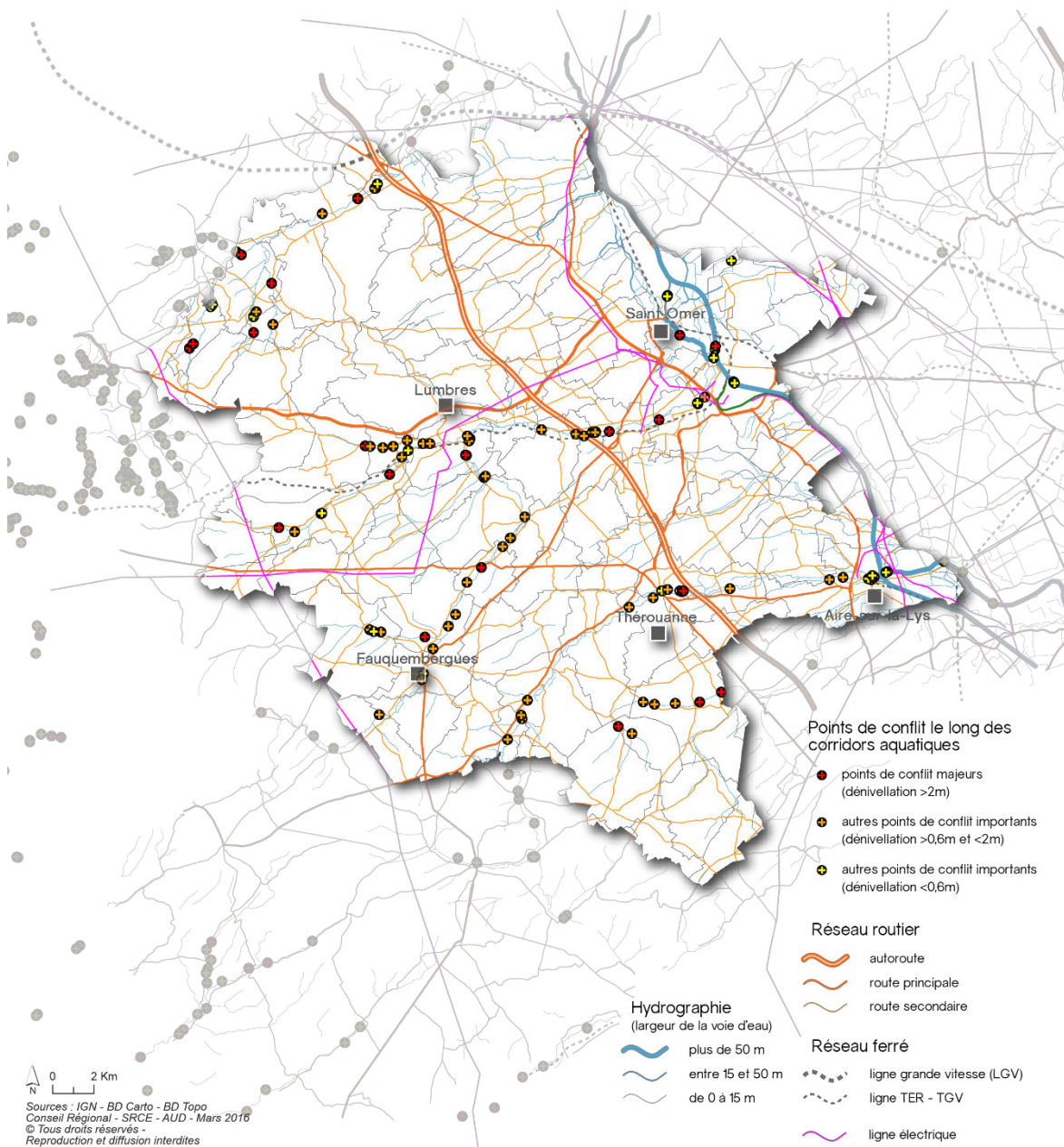
FIGURE 44. ÉLÉMENTS DE FRAGMENTATION DES ESPACES NATURELS
