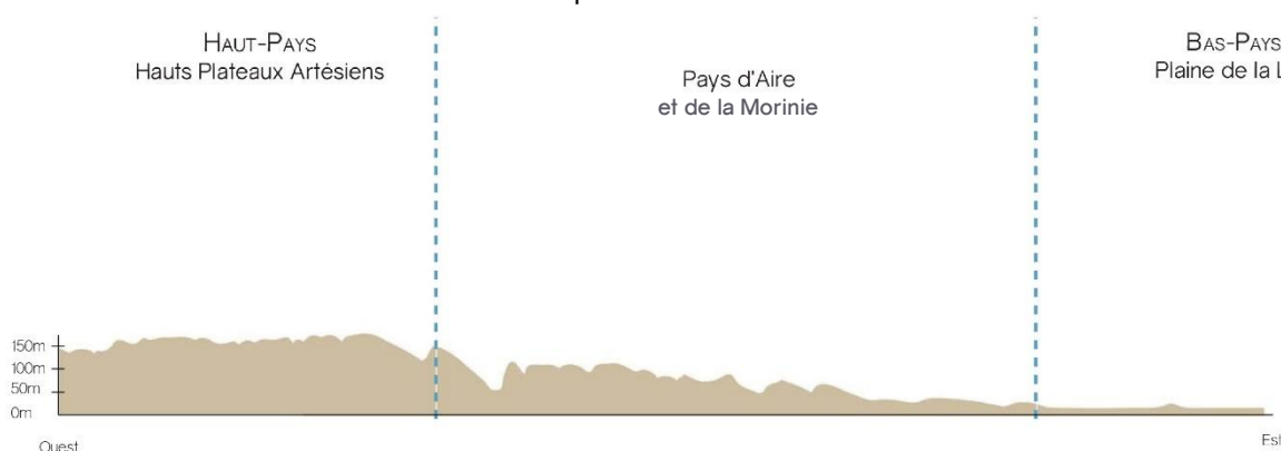
FIGURE 60 COUPE TOPOGRAPHIQUE DU PAYS D'AIRE ET DE LA MORINIE Réalisation AUD-Août 2016
