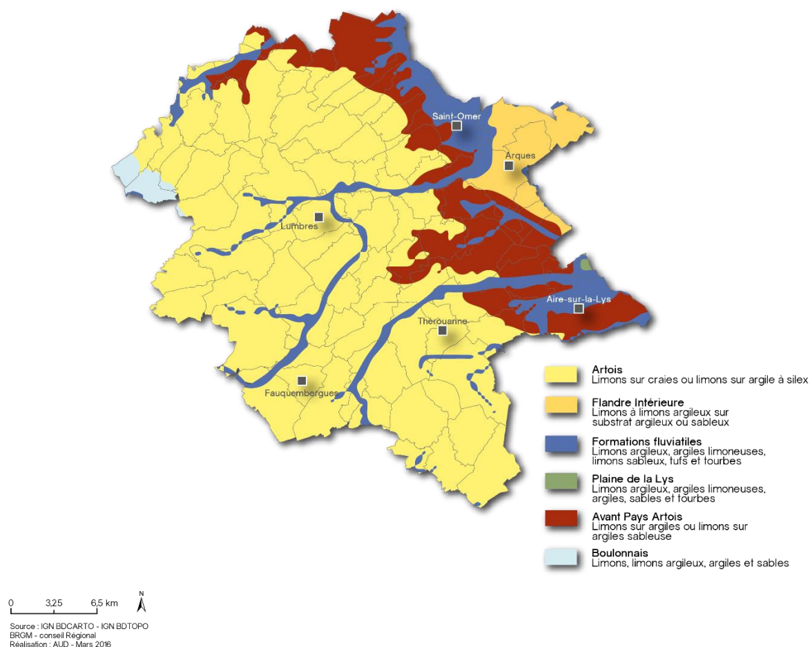
FIGURE 16. FORMATIONS PÉDOLOGIQUES
